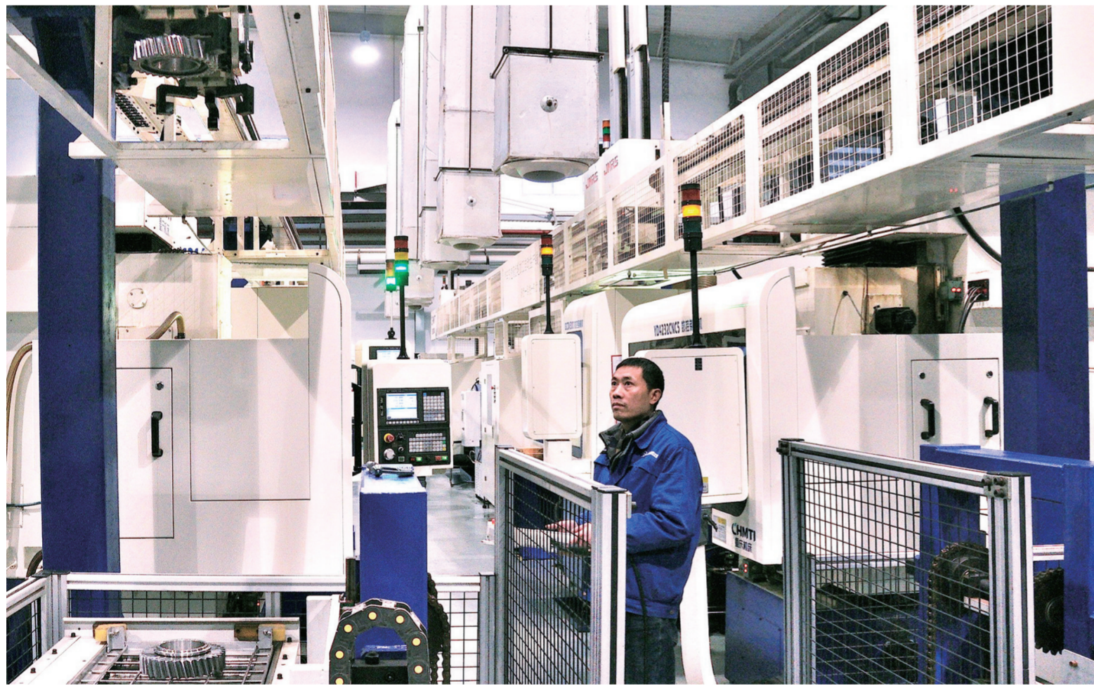
綦齿传动公司一员工在科研项目“复杂修形齿轮精密数控加工关键技术与装备”现场操作机器人卸下已加工完毕的齿轮
