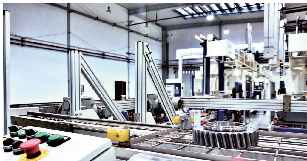
一加工完毕的齿轮在綦齿传动公司科研项目“复杂修形齿轮精密数控加工关键技术与装备”的自动传送架上流动
