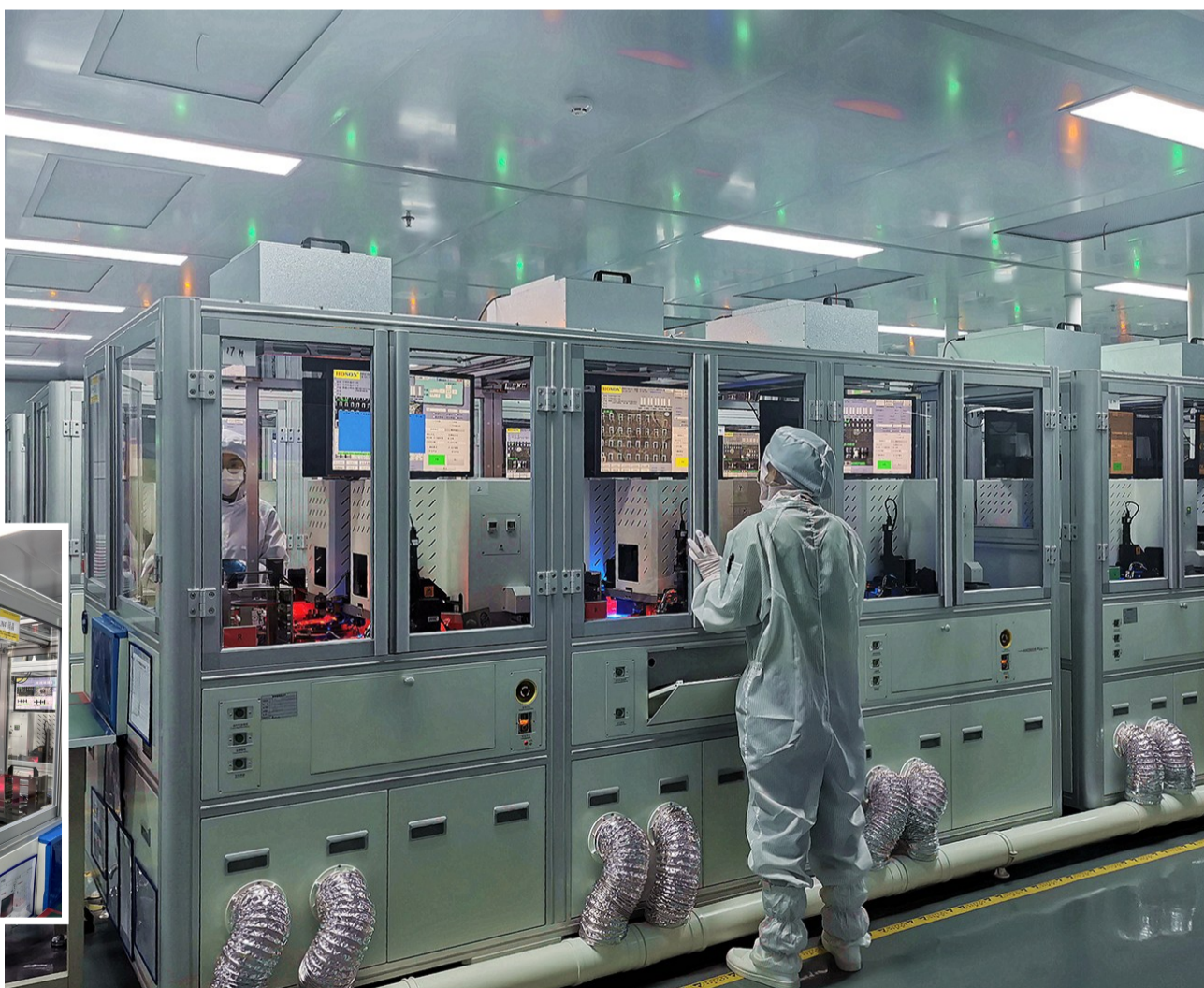
在重庆新视通智能科技有限公司生产车间，工作人员一键操作机器作业。
